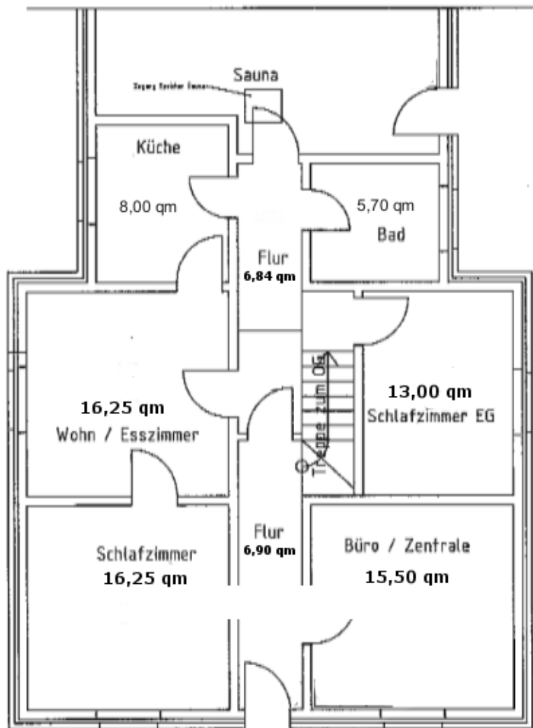
Erdgeschoss
